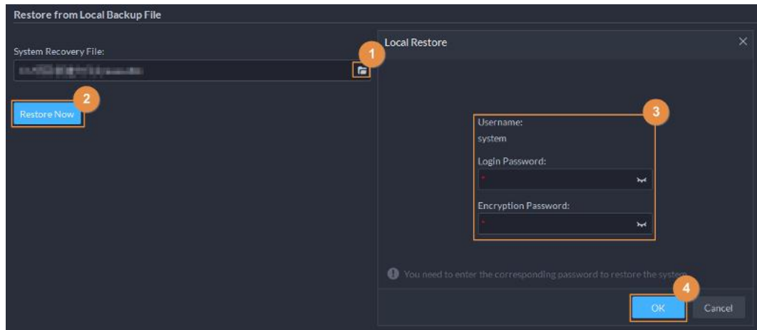
Figure 7-18 Local restore
